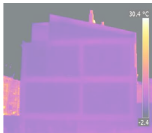
Termografía de vivienda aislada con sistema SATE. Reducción de pérdidas caloríficas, lo que supone un importante ahorro energético en los sistemas de climatización.
